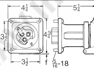
AR Receptacle - Spring Door
